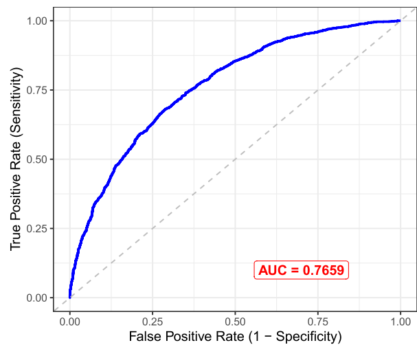
(ج): منحنی ROC برای حالت سوم ( AUC = 0.7659 ).
