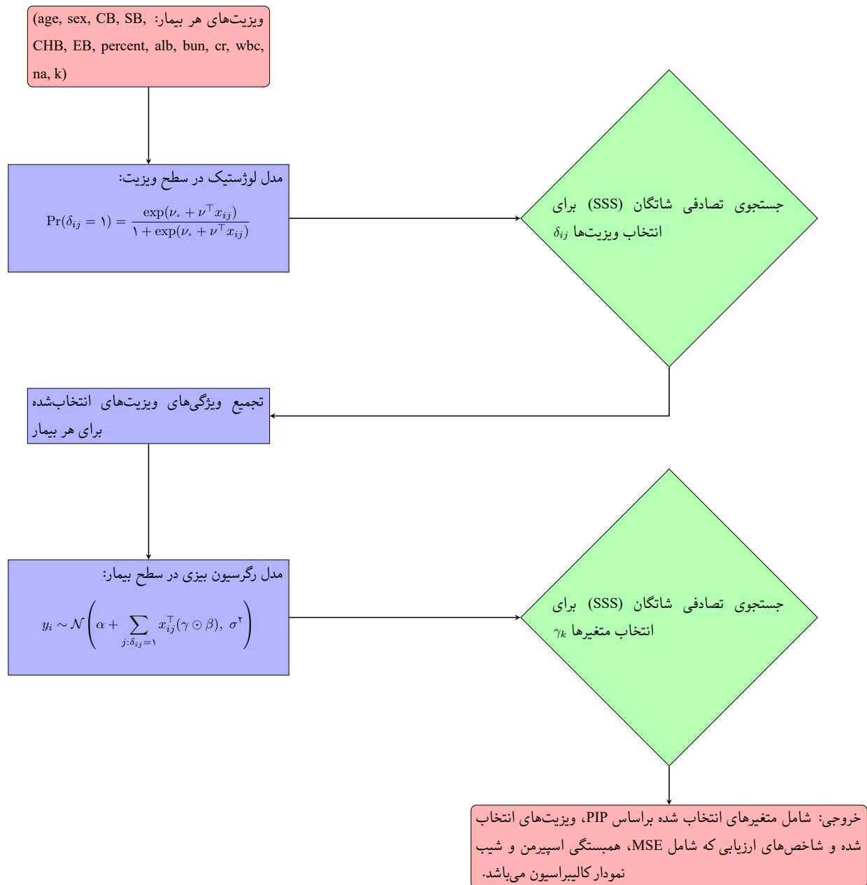
شکل ۴: نمایش الگوریتمی مدل MIR-SSS
