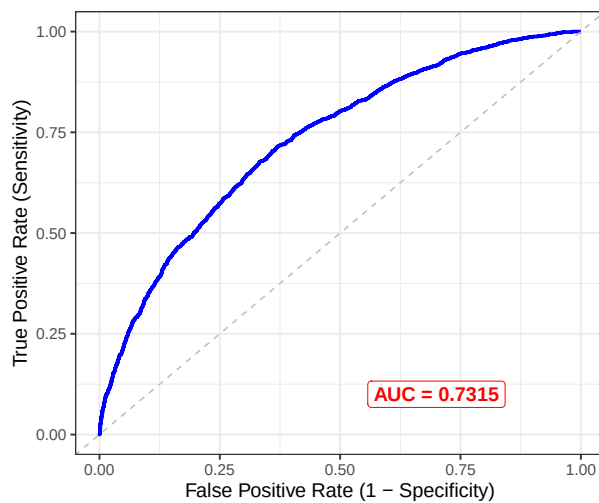
(ب): منحنی ROC برای حالت دوم ( AUC = 0.7315 ).
