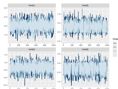
(الف): \beta_1 تا \beta_4
