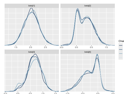
(ت): چگالی \beta_1 تا \beta_4
