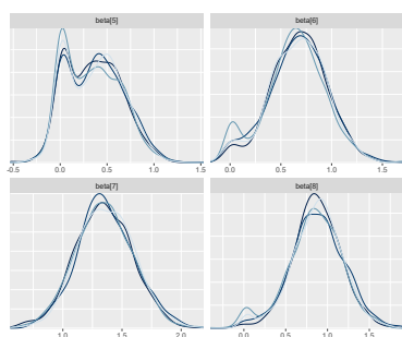
(ث): چگالی \beta_5 تا \beta_8
