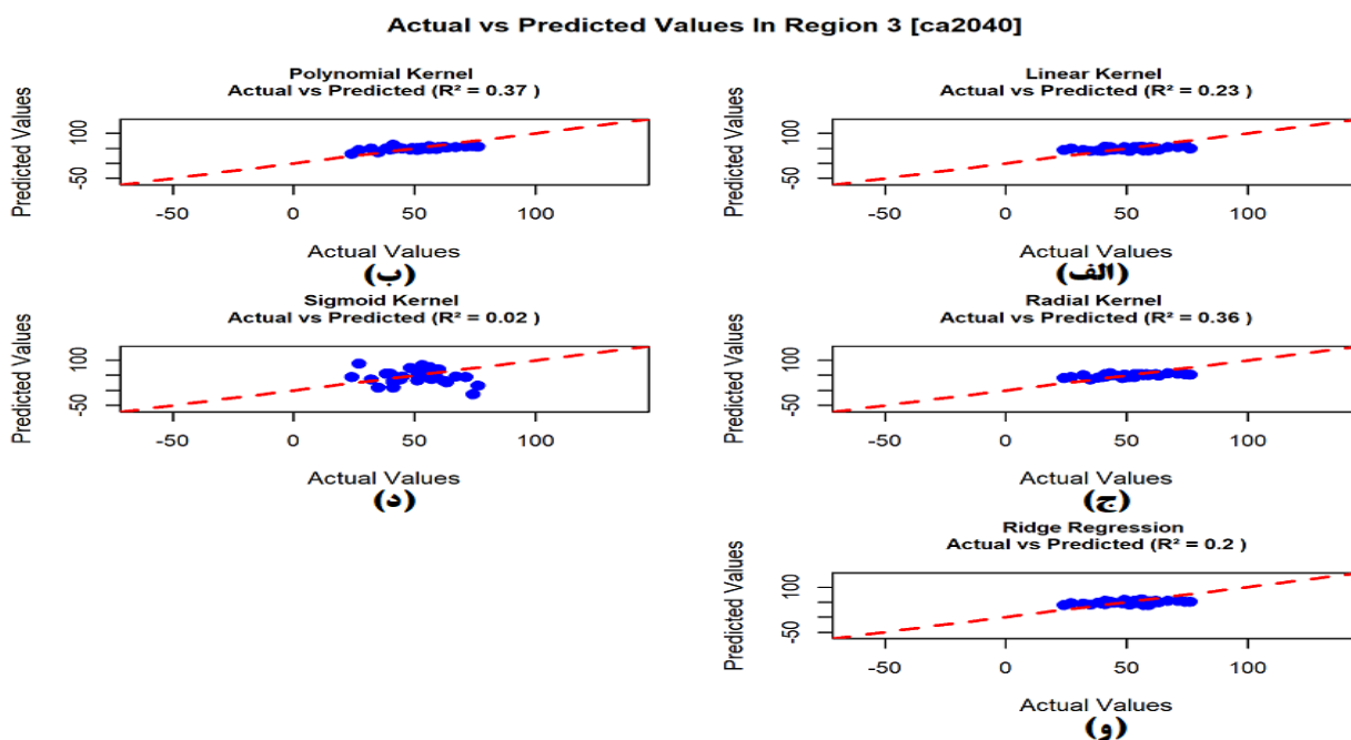
شکل ۷: نمودار مقادیر واقعی در برابر مقادیر پیش‌بینی شده برای چهار هسته بردار پشتیبان و رگرسیون ریبج در منطقه ۳ در ca2040 : (الف) هسته خطی، (ب) هسته چندجمله‌ای، (ج) هسته شعاعی، (د) هسته سیگموئید، (و) رگرسیون ریبج.
