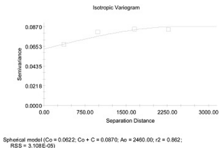
شکل ۱۸. واریوگرام طلا در منطقه مورد مطالعه
