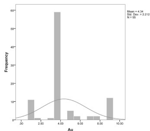
شکل ۶. نمودار فراوانی متغیر طلا بر روی داده‌های خام
