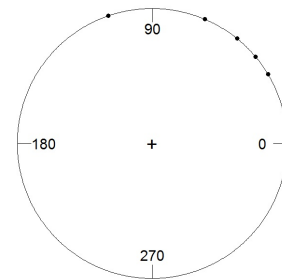
شکل ۹. نمودار پراکنش داده‌های دایره‌ای در نرم‌افزار R
