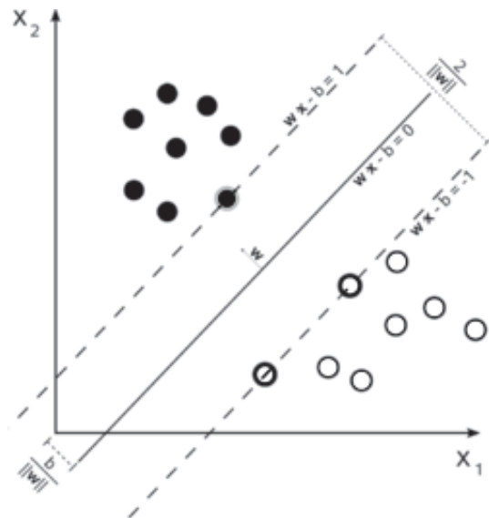
شکل ۱۰: حاشیه خطوط رده‌بند در ماشین بردار پشتیبان
