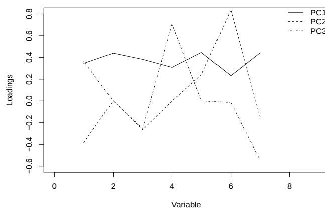
شکل ۵. نمودار مقادیر بار حاصل از رویکرد ROSPCA ( k=3 ، \lambda=0.54 و \alpha=0.5 ).
