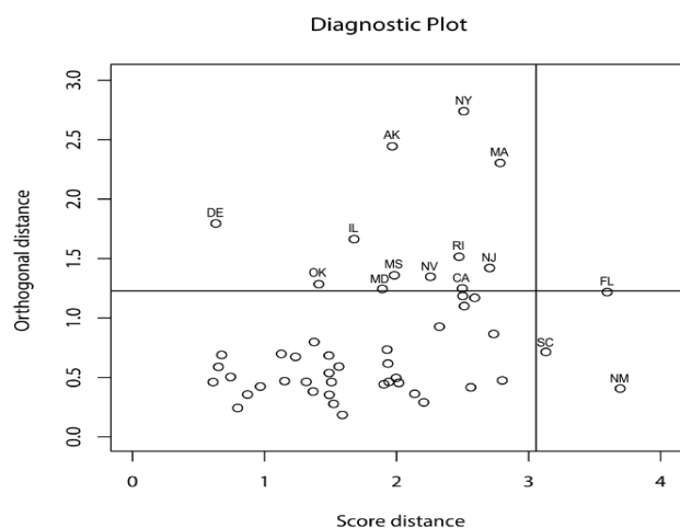
شکل ۴. نمودار تشخیصی مربوط به رویکرد ROSPCA ( k=3 ، \alpha=0.5 و \lambda=0.54 ).
