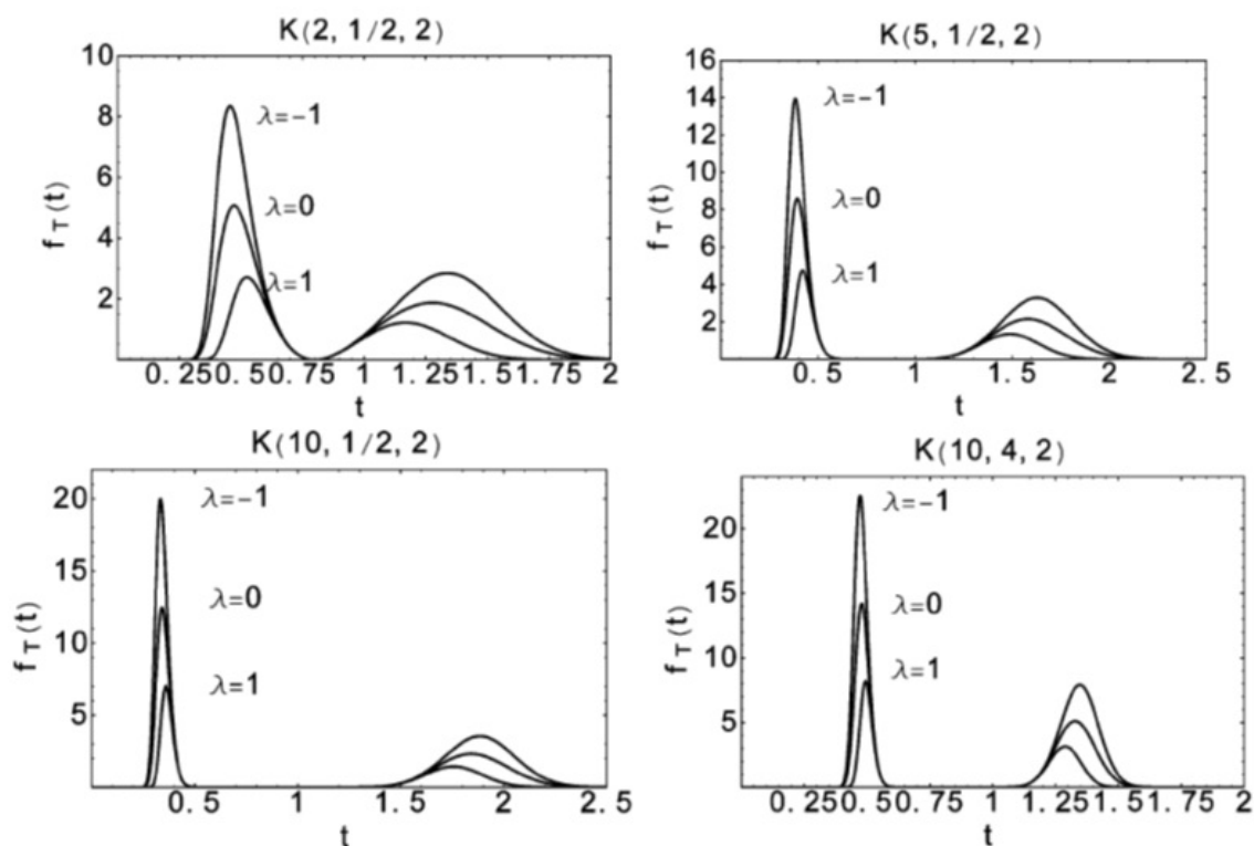
شکل ۶: نمودارهای چگالی توزیع GBS'' حاصل از توزیع کاتز-نوع KT(q, r, s) برای \alpha = 0.5 و \beta = 0.8 و q و r و s تعیین شده (KT(q, r, s))
