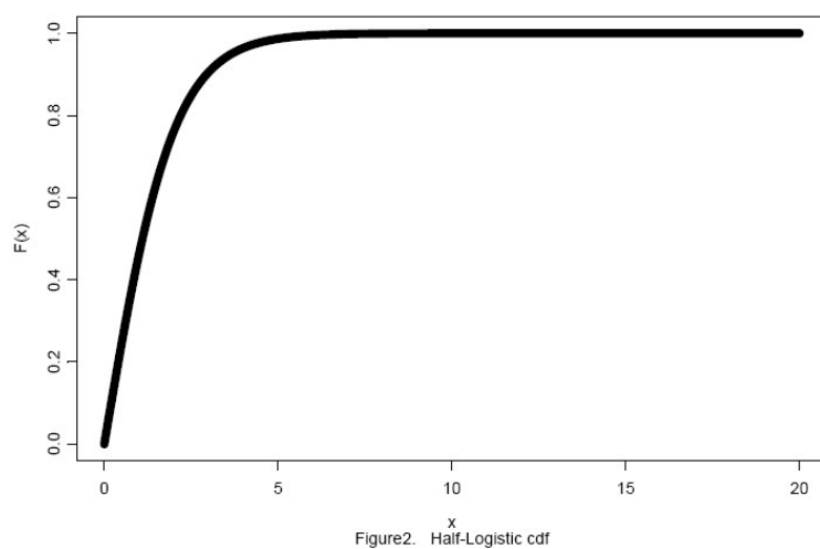
شکل ۲: تابع توزیع تجمعی نیمه لجستیک
