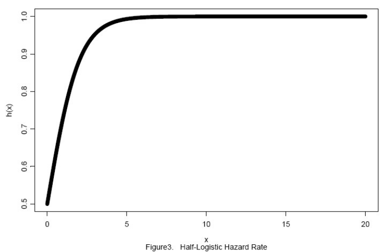
شکل ۳: نمودار تابع خطر h(x)
